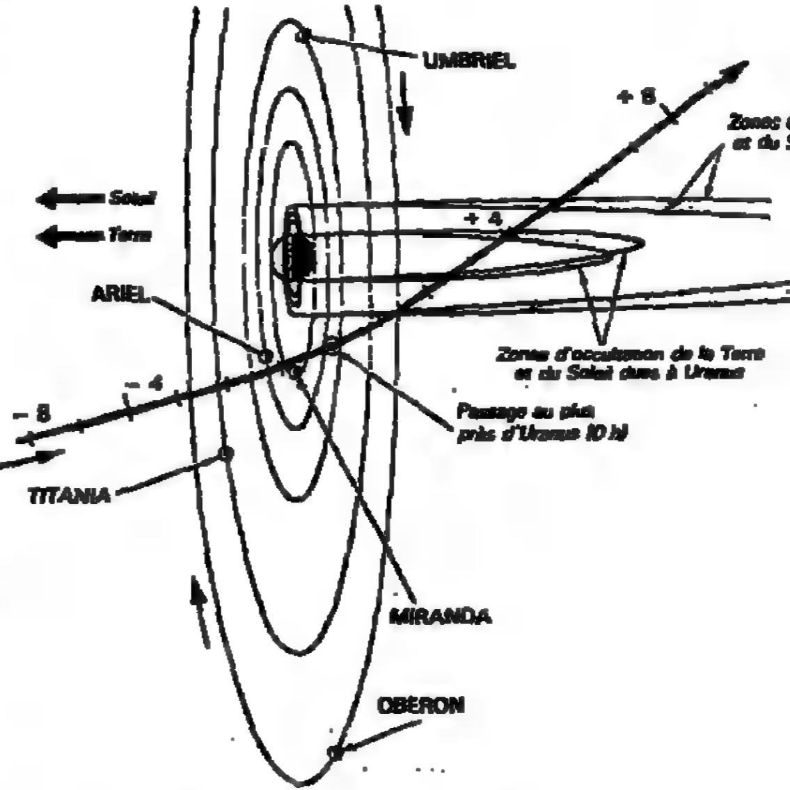
La figure représente Uranus, ses anneaux, ses satellites et la trajectoire de Voyager-2 — graduée en heures à partir du point de plus faible approche (vendredi 24 janvier, à 19 heures). La sonde arrive du côté du pôle Sud, puis passe derrière l'hémisphère Nord, en traversant les ombres portées par la planète et ses anneaux.
